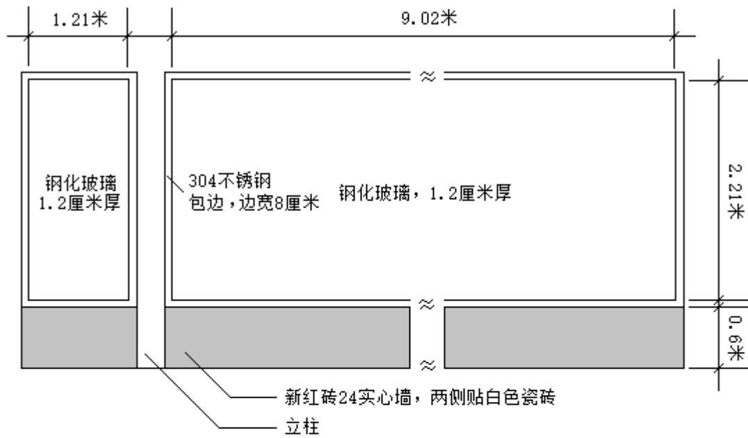
隔断侧面图 (局部):
